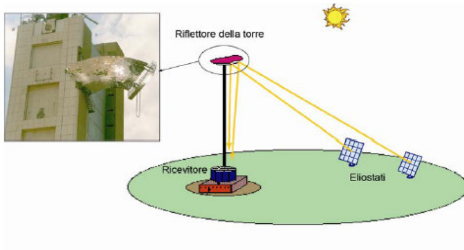
Figura 10 – Schema di un impianto a torre con ricevitore a terra
