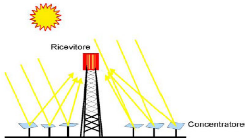
Figura 6 – Schema di principio di un sistema torre
