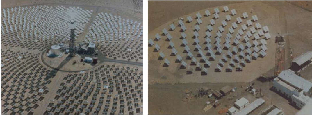
Figura 7 – Differenti disposizioni degli eliostati in un sistema a torre.
