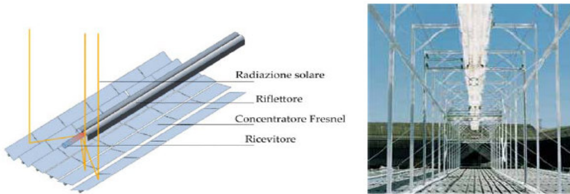
Figura 18 – Il sistema Fresnel
