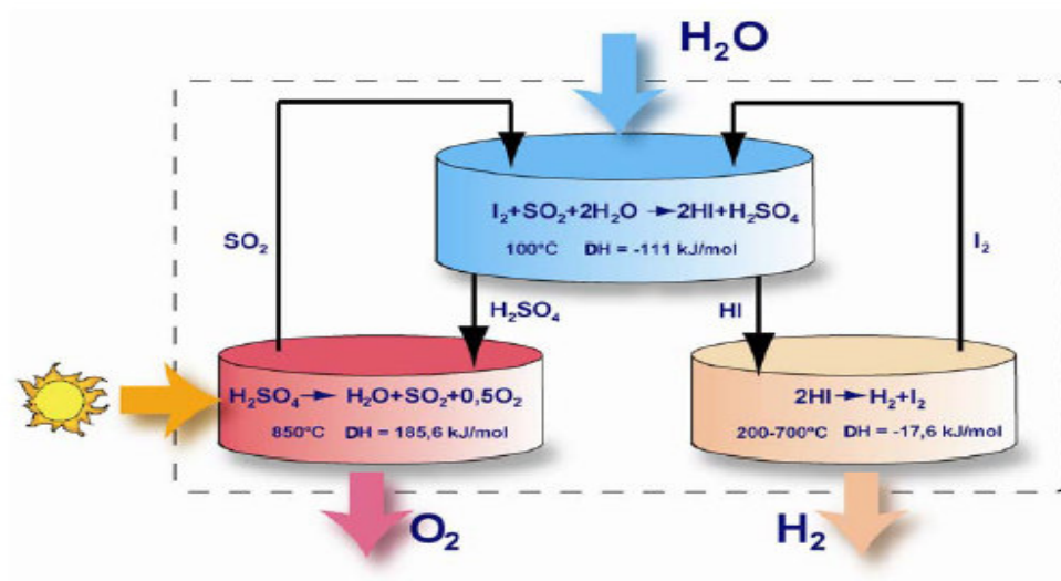
Figura 20 – Schema del processo zolfo-iodio
