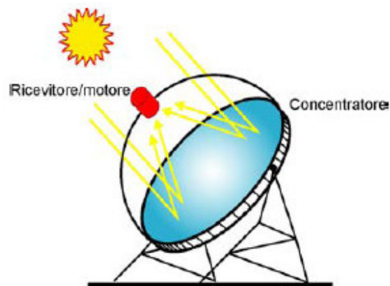
Figura 3 – Schema di principio di un disco parabolico
