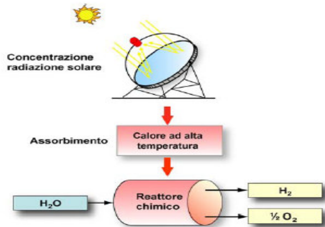
Figura 19 – Schema della produzione di idrogeno
