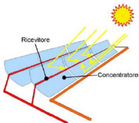
Figura 11 – Schema di principio di un sistema a concentratori parabolici lineari.
