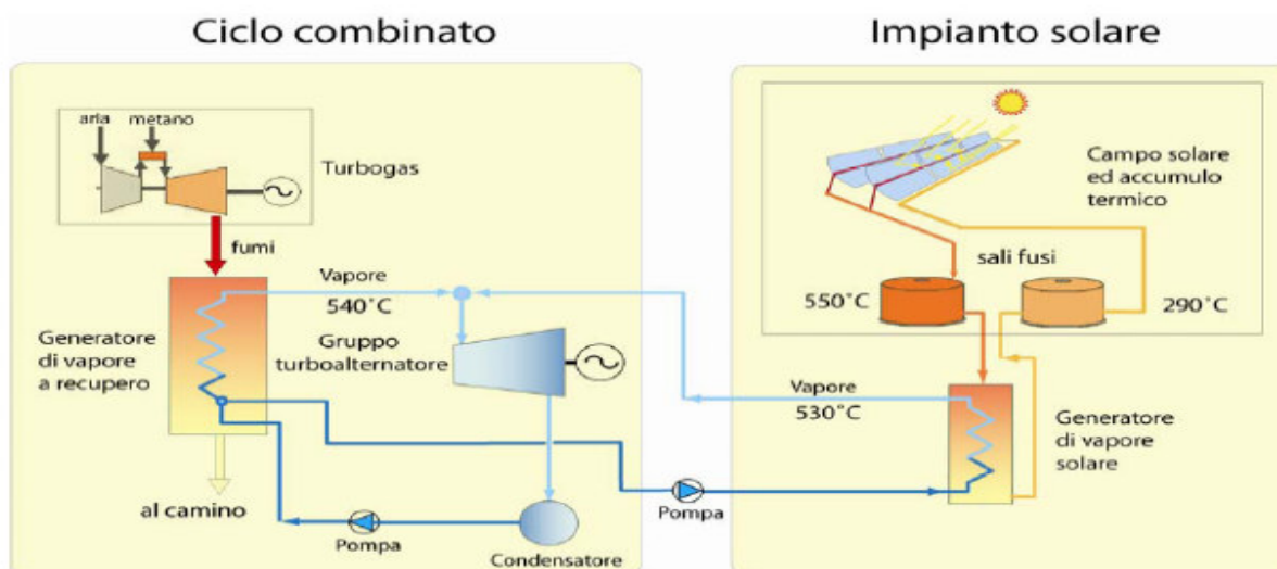
Figura 17 – Schema di massima del progetto "Archimede"
